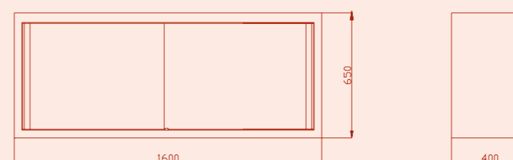
Beispiel: Wandhängeschränk mit Schiebetüren, 1600x400x650mm
